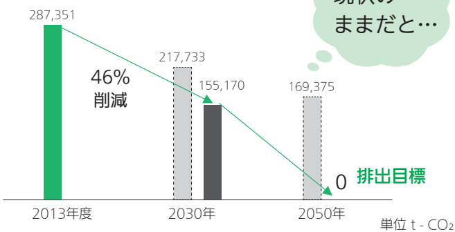
芳賀町のCO 2 排出削減目標
