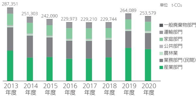
芳賀町のCO 2 排出量の推移
