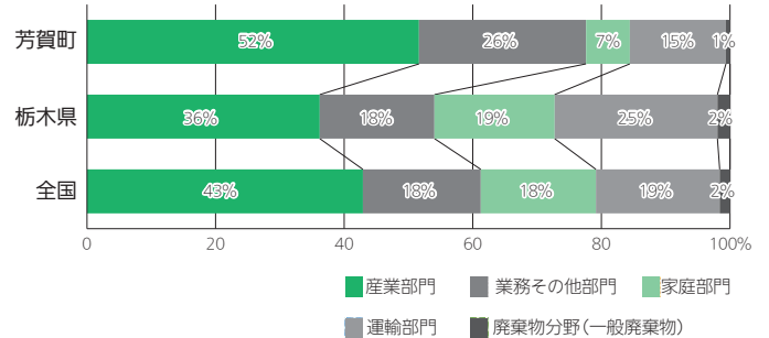
CO 2 部門別排出量割合の芳賀町・県・国の比較
